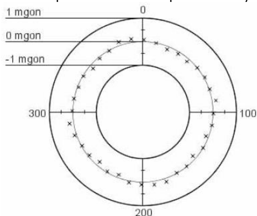
Рис 4 – Дисперсия измерения горизонтального угла TPM. ISO 17123-3 (n = 36): 0.14мгон
